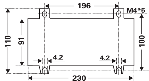
图2:底部平面图尺寸
