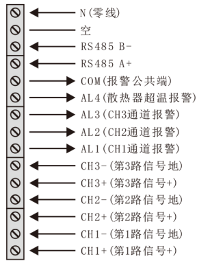
接线端子说明 (SCR横放, 端子朝右)
