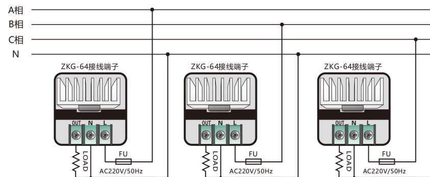
三相接线图:
