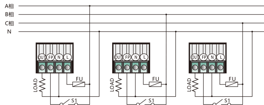
三相接线图：
